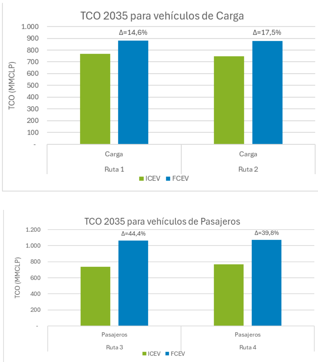
Figura 6-46: TCO por ruta y tipo de vehículo al año 2035 como inicio de operación
