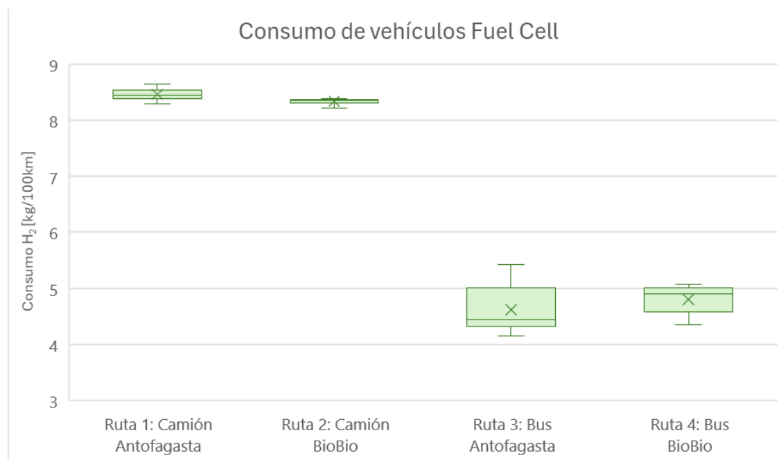
Figura 6-51: Variabilidad del rendimiento energético de los vehículos con Fuel Cell.
