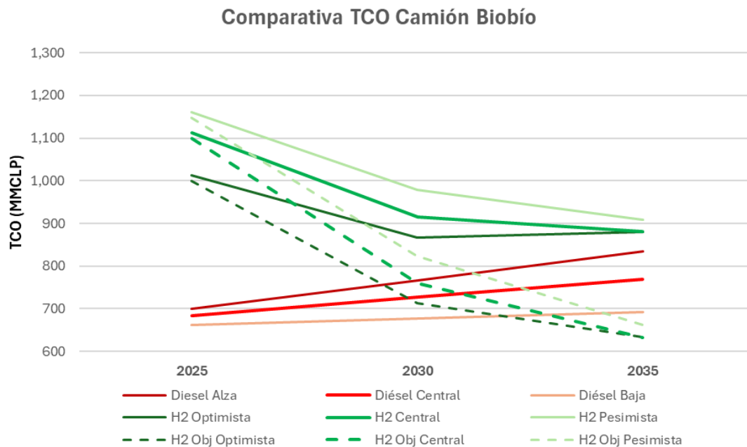
Figura 6-53: Comparativa TCO Recorrido 2 en función de los costos de los energéticos y de inversión
