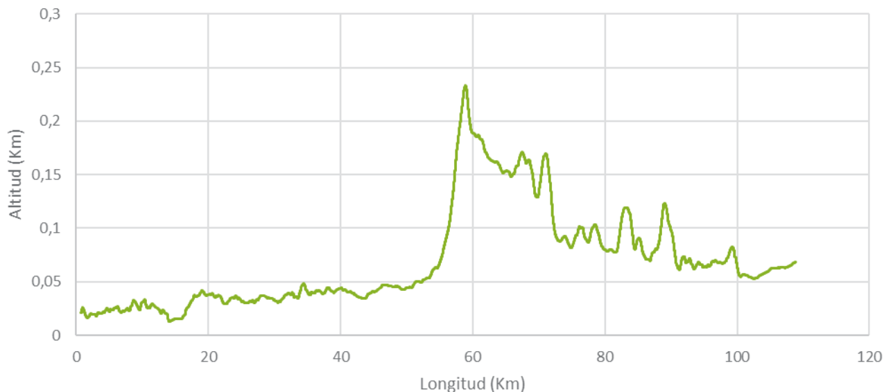
Figura 9-32: Perfil de Elevación Ruta 156 (Media móvil de período 100).
