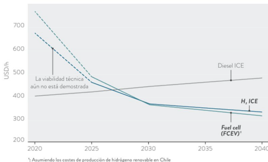
Figura 3-19: Evolución de Costos Totales para CAEX (En base a camión de 300 toneladas a cielo abierto)
