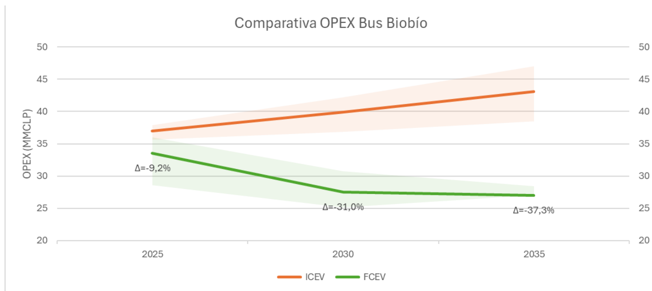
Figura 6-59: Comparativa OPEX de la Ruta 4.
