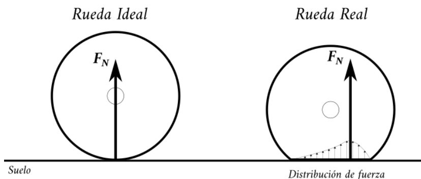
Figura 6-26: Comparativa de fuerzas aplicadas en una rueda ideal y una real.
