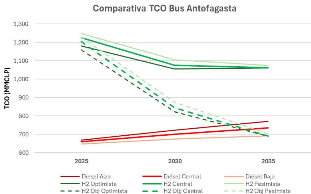
Figura 6-54: Comparativa TCO Recorrido 3 en función de los costos de los energéticos y de inversión
