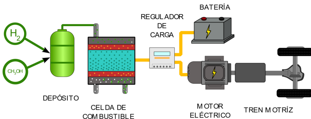
Figura 2-5: Componentes principales de un Vehículo Eléctrico con Pila de Combustible alimentado con metanol o con hidrógeno (FCEV)
