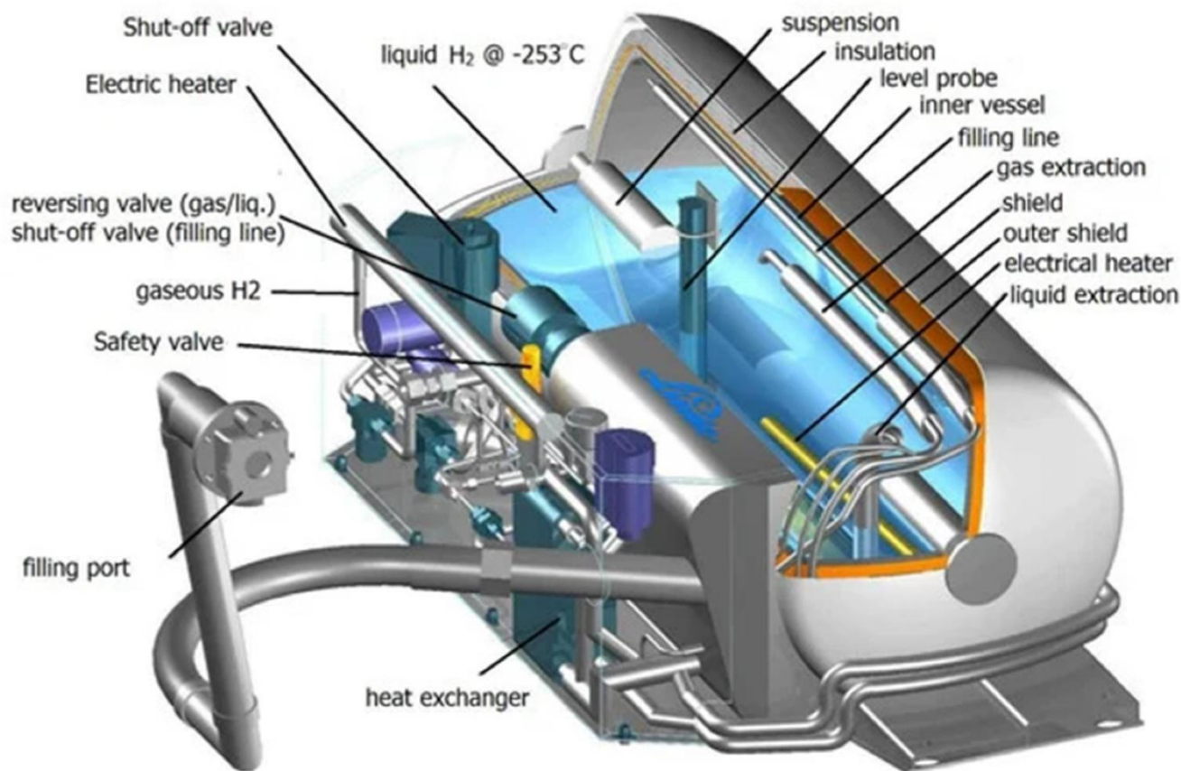
Figura 2-10: Esquema interior de estanque de almacenamiento de hidrógeno líquido
