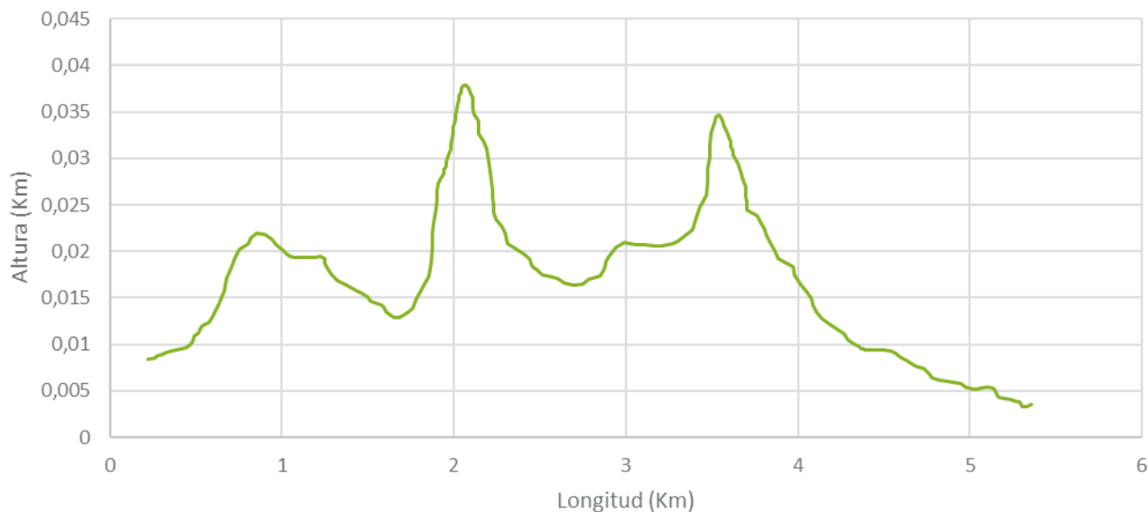
Figura 9-31: Perfil de Elevación Ruta 154 (Media móvil de período 10).
