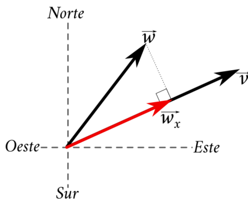
Figura 6-30: Esquema de cálculo de la proyección de la velocidad del viento.
