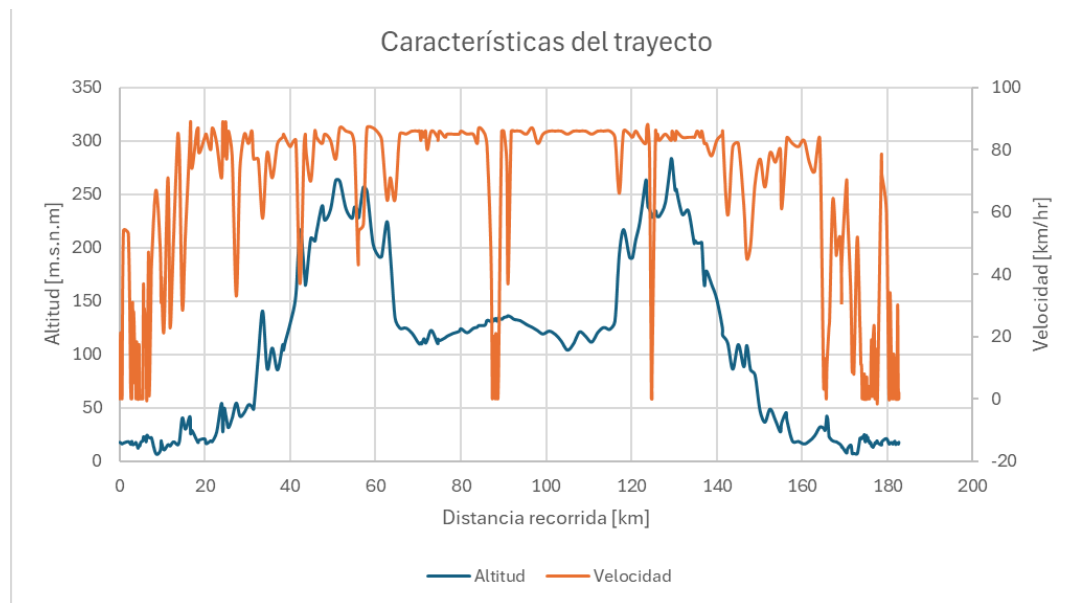
Figura 6-38: Características del trayecto de la Ruta 2 de transporte de carga.
