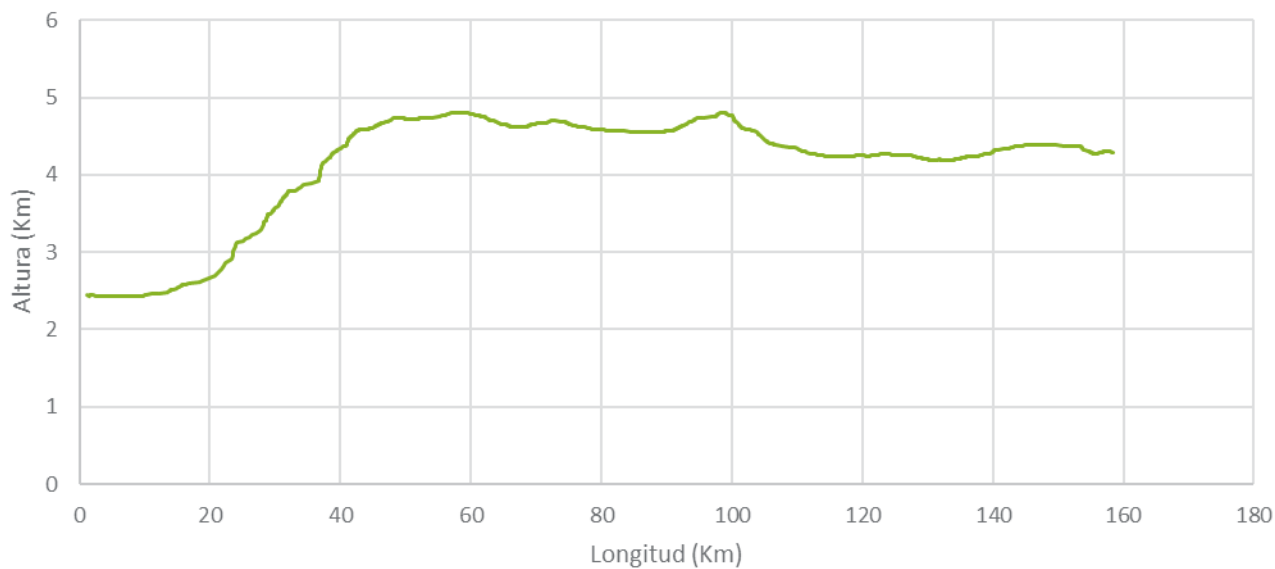
Figura 9-9: Perfil de Elevación Ruta 27 (Media móvil de período 10).
