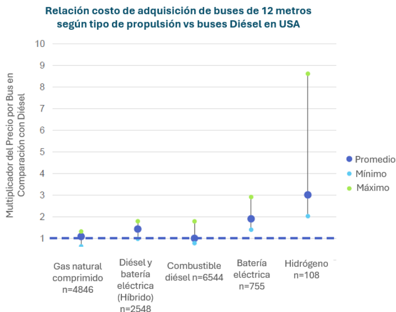
Figura 3-4: Relación costo de adquisición de buses de 12 metros según tipo de propulsión vs buses Diésel en USA
