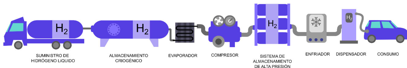
Figura 2-17: Estación de carga de hidrógeno líquido
