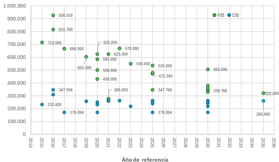
Figura 3-5: Costo de adquisición de buses a hidrógeno vs buses Diésel según literatura (EUR)
