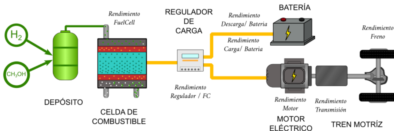
Figura 6-28: Modelo de un vehículo con celda de combustible
