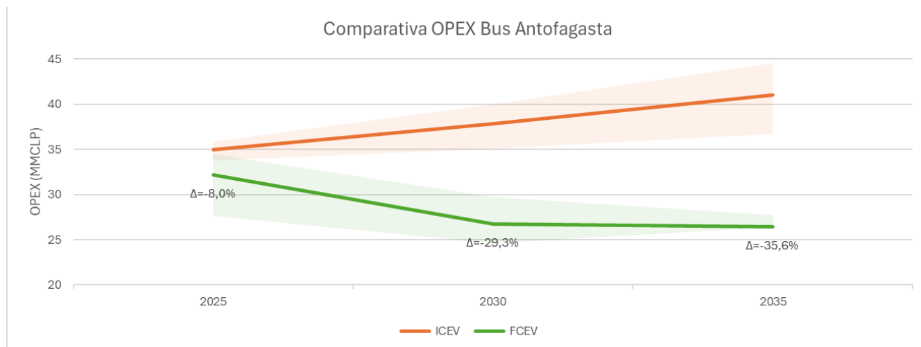
Figura 6-58: Comparativa OPEX de la Ruta 3.
