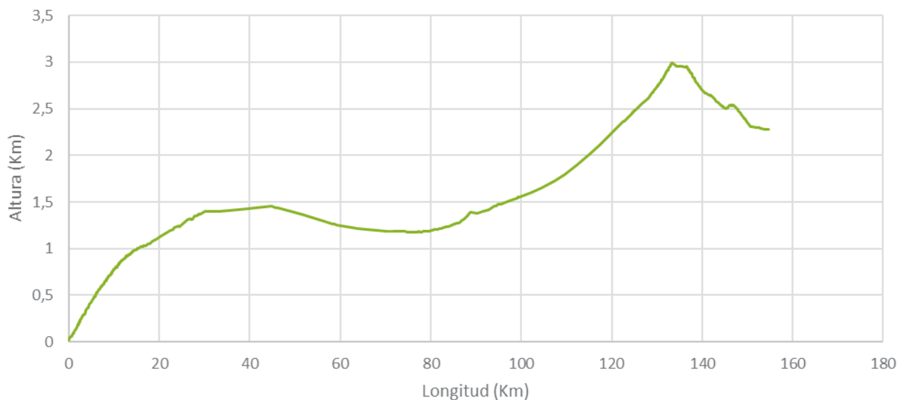
Figura 9-6: Perfil de Elevación Ruta 24.
