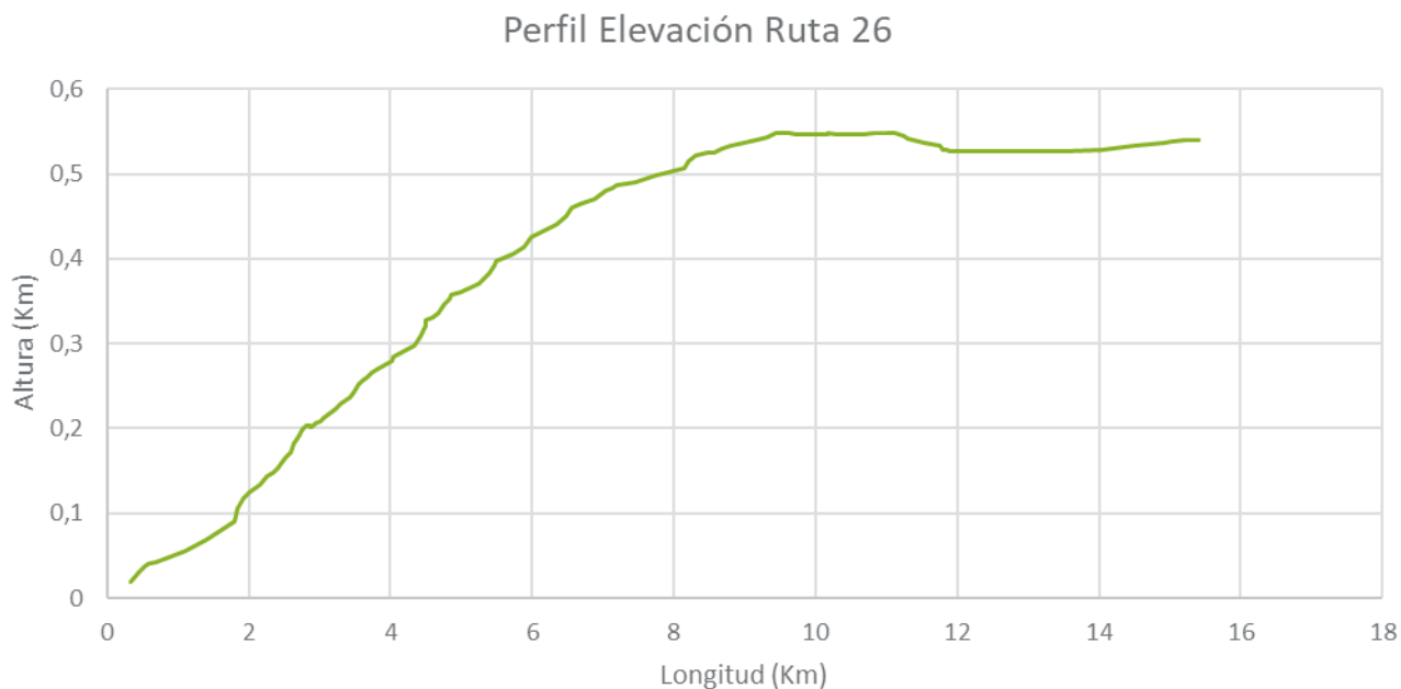
Figura 9-8: Perfil de Elevación Ruta 26 (Media móvil de período 3)
