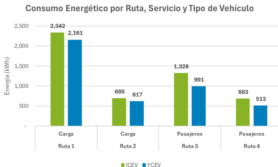
Figura 6-43: Consumo de energía por ruta y tipo de vehículo
