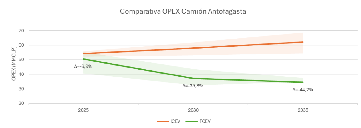
Figura 6-56: Comparativa OPEX de la Ruta 1.
