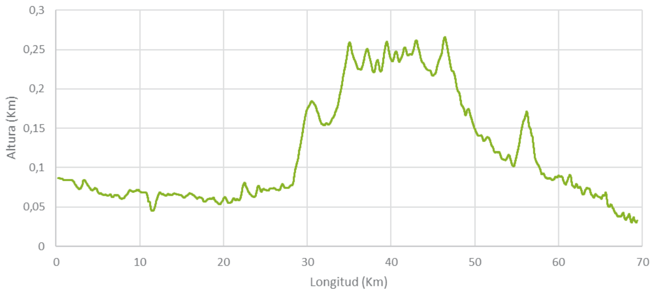
Figura 9-12: Perfil de Elevación Ruta N-48-O (Media móvil de período 50).
