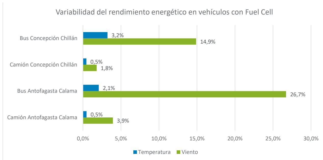
Figura 6-49: Variabilidad del rendimiento de los vehículos con Fuel Cell en función de las condiciones meteorológicas
