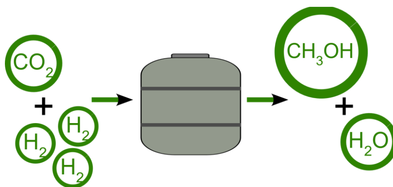
Figura 2-2: Producción de metanol
