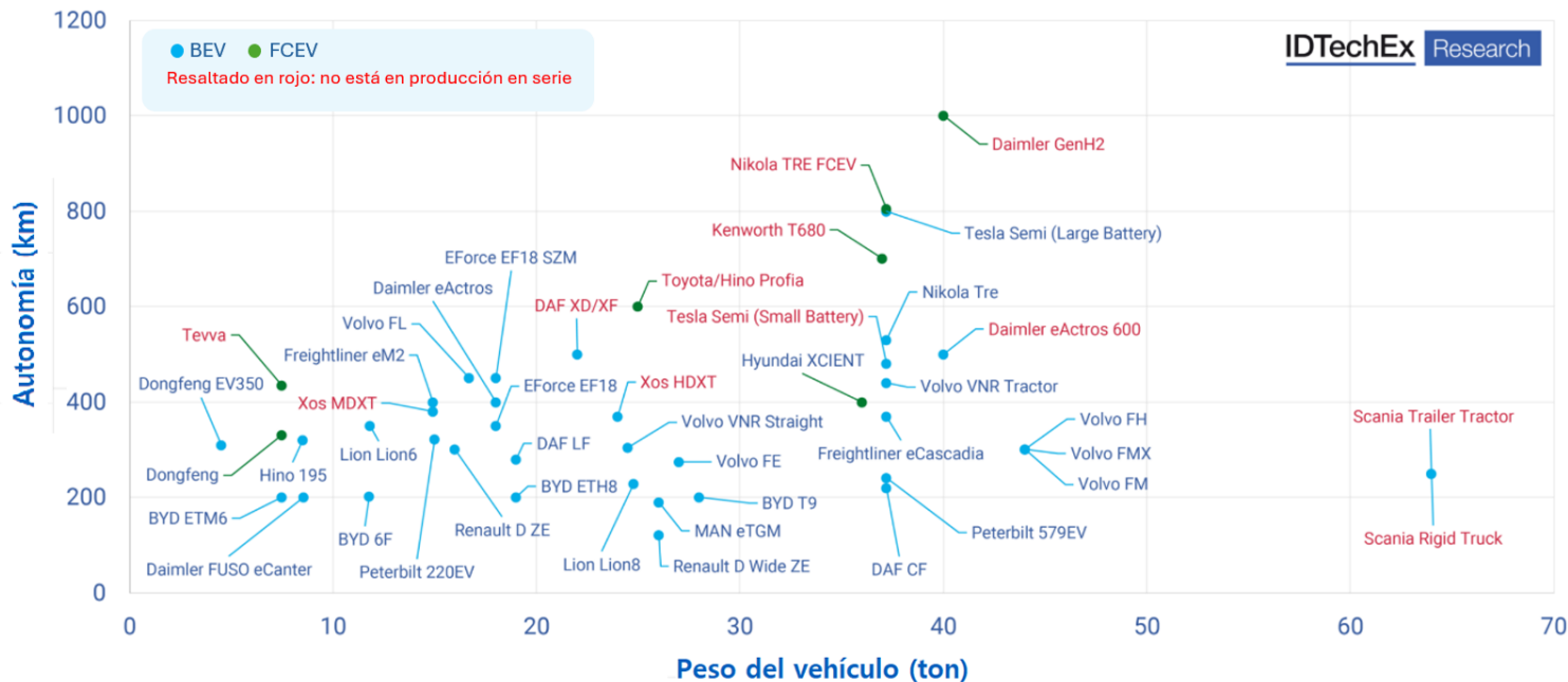
Figura 3-17: Autonomía de camiones de cero emisiones según peso del vehículo y alcance
