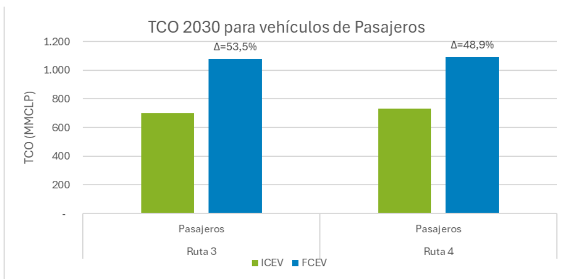
Figura 6-45: TCO por ruta y tipo de vehículo al año 2030 como inicio de operación
