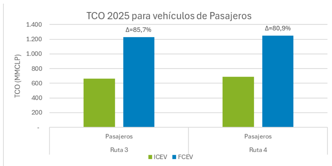
Figura 6-44: TCO por ruta y tipo de vehículo al año 2025 como inicio de operación
