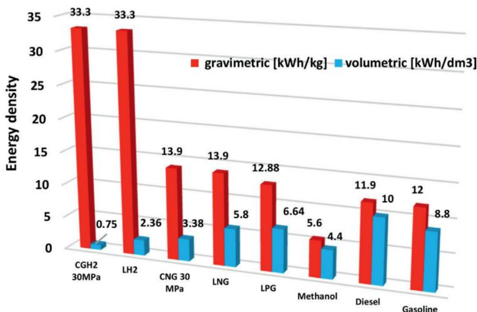
Figura 2-7: Densidad energética por unidad de masa y volumen de varios combustibles químicos
