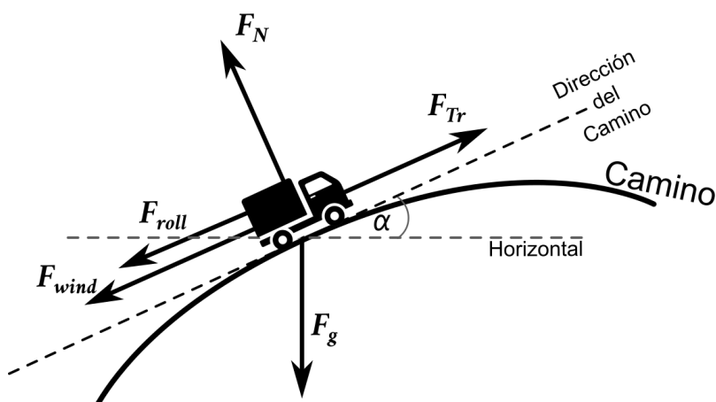
Figura 6-24: Diagrama de cuerpo libre: Fuerzas actuando en el vehículo.
