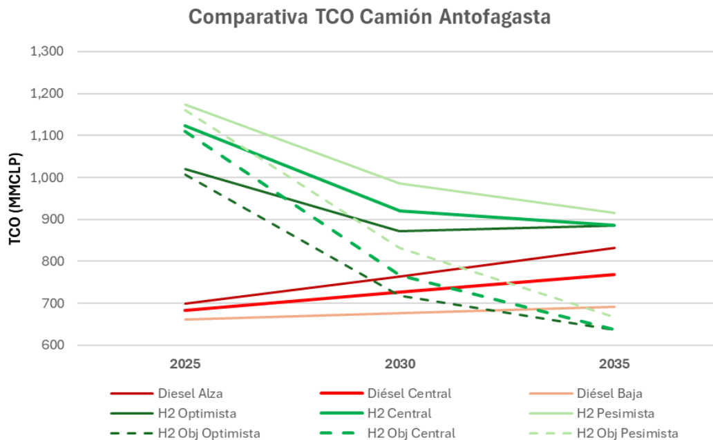
Figura 6-52: Comparativa TCO Recorrido 1 en función de los costos de los energéticos y de inversión
