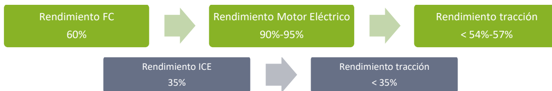
Figura 2-4: Comparativa rendimientos ICE vs FCEV
