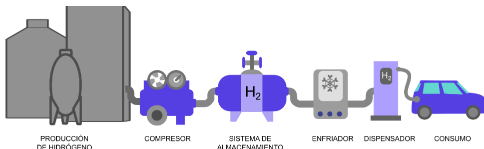
Figura 2-16: Estación de carga de hidrógeno gaseoso
