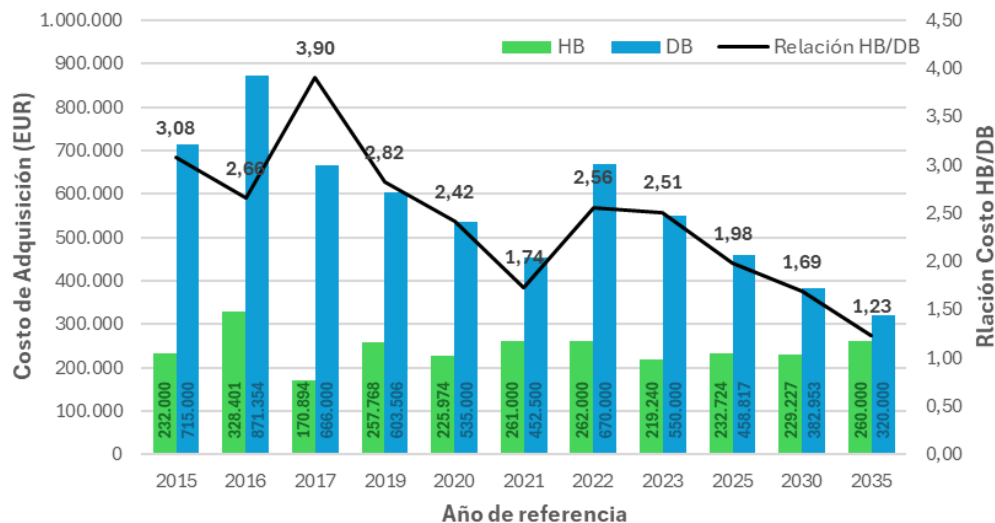
Figura 3-7: Costo de adquisición promedio buses a hidrógeno vs buses Diésel según literatura (EUR)
