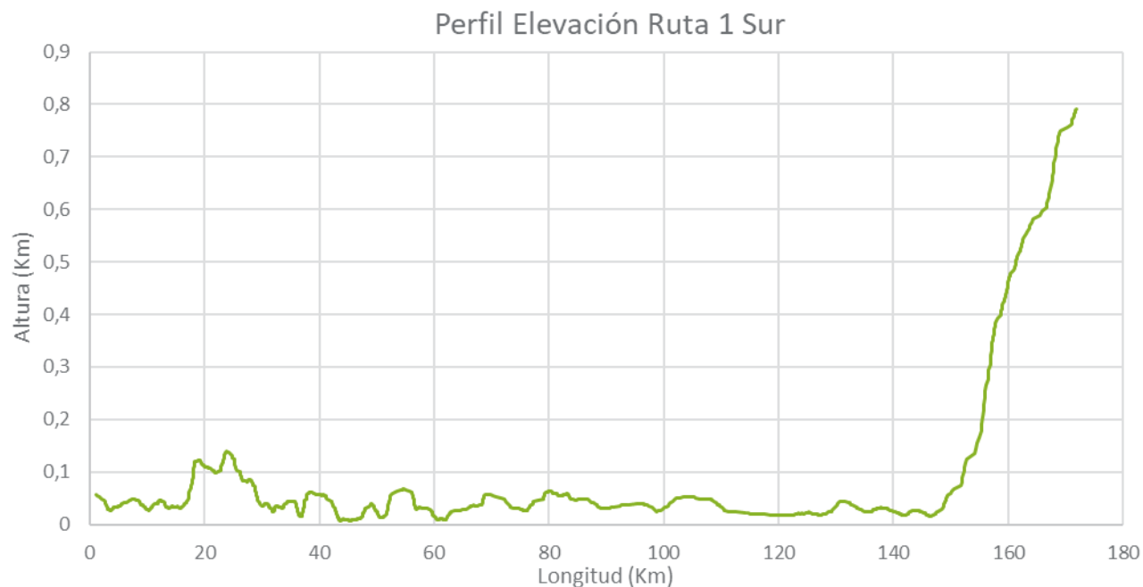
Figura 9-2: Perfil de Elevación Ruta 1 Tramo Sur (Media móvil de período 20).
