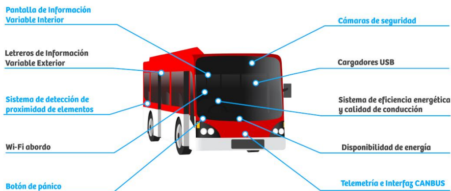
Figura 5-6: Principales elementos y sistemas tecnológicos buses estándar RED
