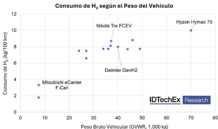
Figura 3-18: Consumo de Hidrógeno según peso de vehículo, camiones FCEV
