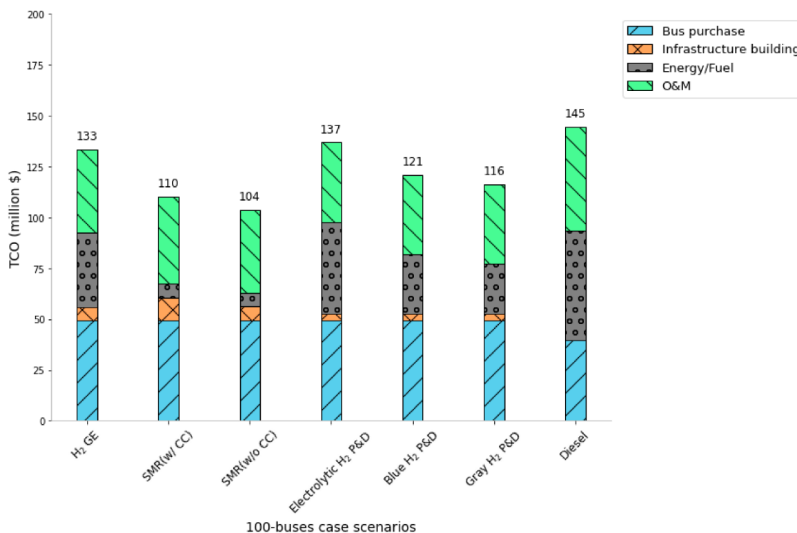
Figura 2-29: TCO para caso estudio de flota de 100 buses en New Jersey, Estados Unidos (2028)
