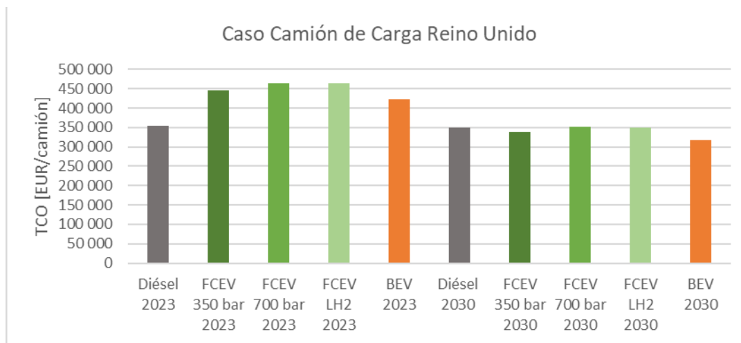
Figura 2-27: Costos Totales de Propiedad (TCO) para caso de estudio de flota de camiones en Inglaterra
