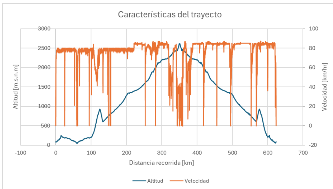
Figura 6-36: Características del trayecto de la Ruta 1 de transporte de carga
