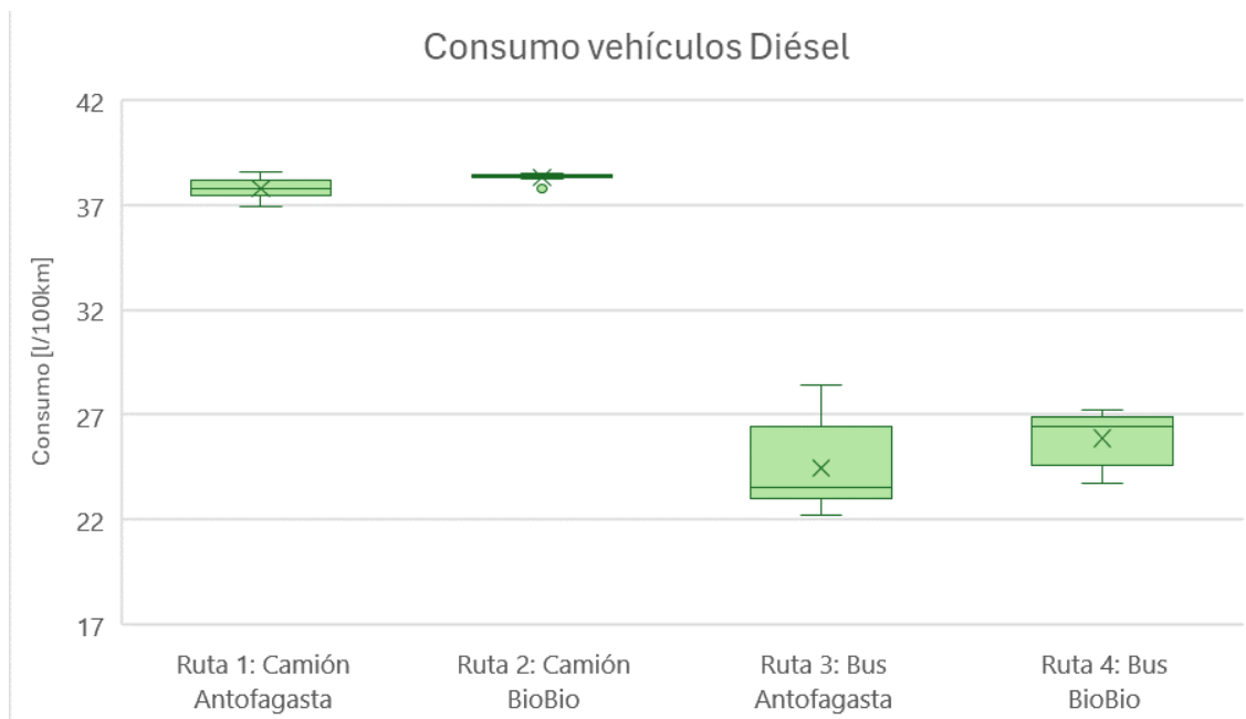
Figura 6-50: Variabilidad del rendimiento energético de los vehículos Diesel.
