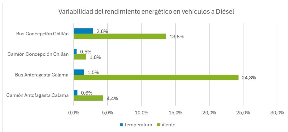
Figura 6-48: Variabilidad del rendimiento de los vehículos diésel en función de las condiciones meteorológicas
