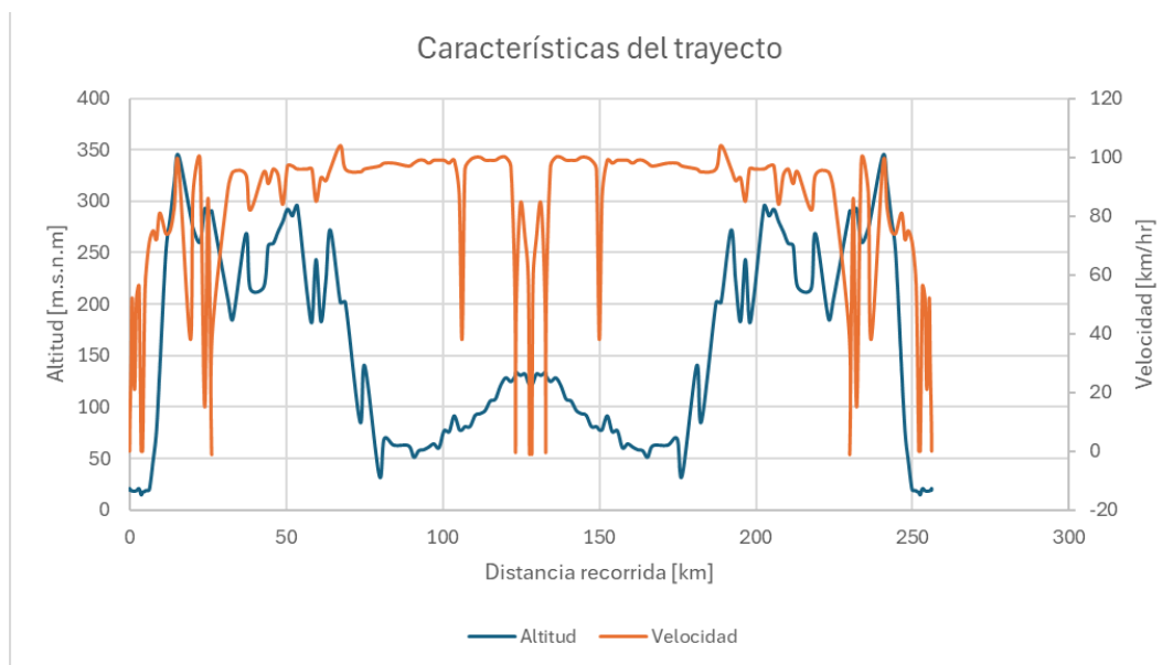
Figura 6-42: Características del trayecto de la Ruta 4 de transporte de pasajeros.
