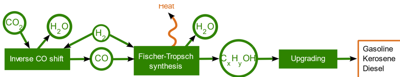
Figura 2-3: Producción de e-diésel vía Proceso Fischer-Tropsch
