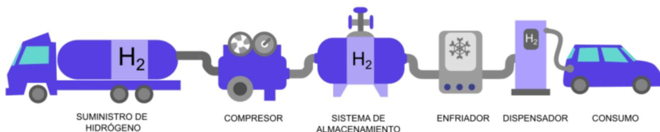
Figura 2-13: Representación esquemática de una estación de carga
