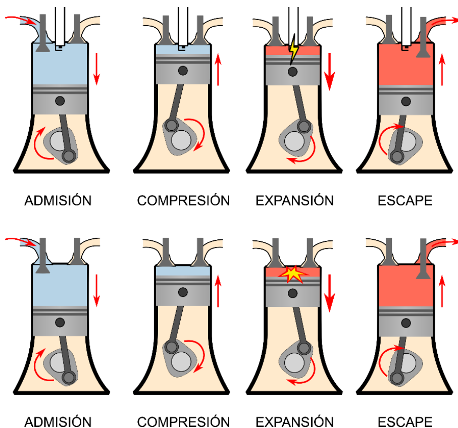
Figura 2-12: Esquema de funcionamiento de un ICE. Arriba: con Ciclo Otto. Abajo: con Ciclo Diésel
