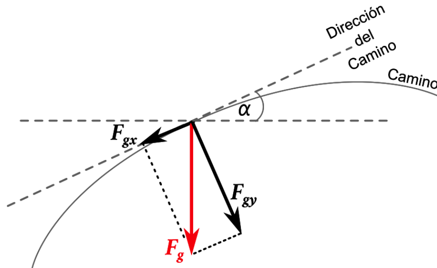
Figura 6-25: Descomposición vectorial de la fuerza de gravedad.
