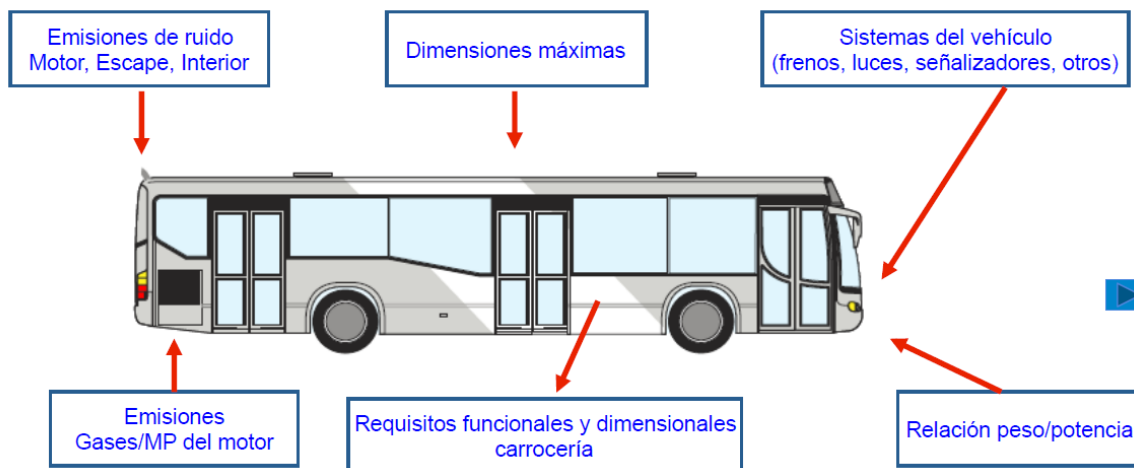
Figura 5-7: Principales ámbitos que contempla la certificación de un bus urbano Sistema RED
