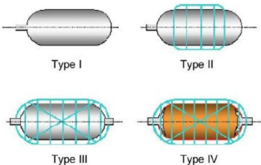
Figura 2-9: Tipos de tanques de hidrógeno
