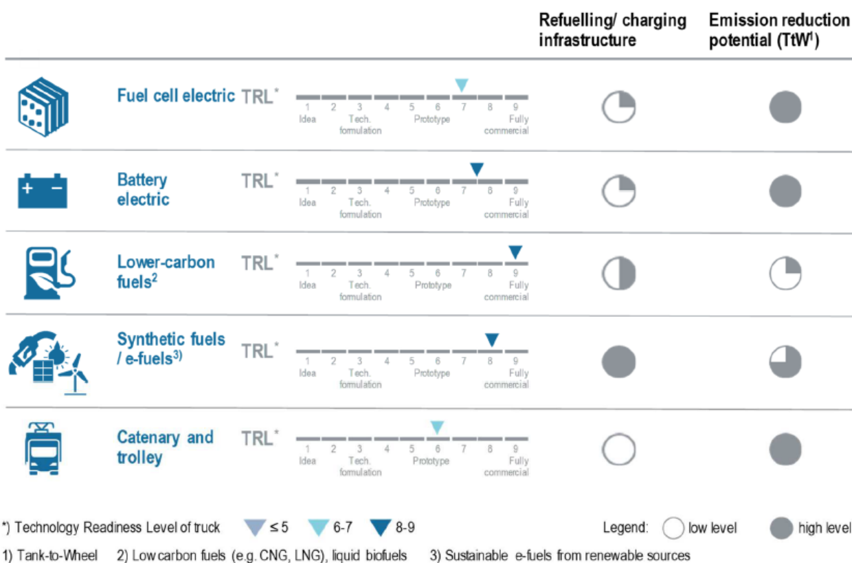
Figura 2-1: Comparativa de tecnologías de propulsión alternativas para camiones pesados
