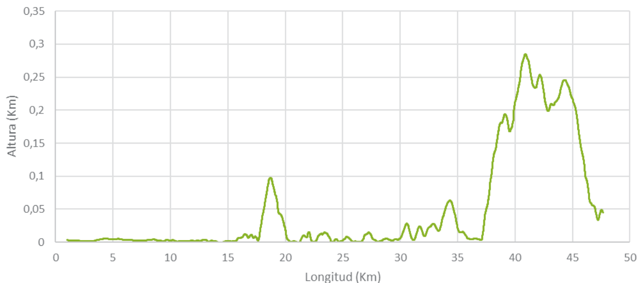
Perfil Elevación Ruta P-20
