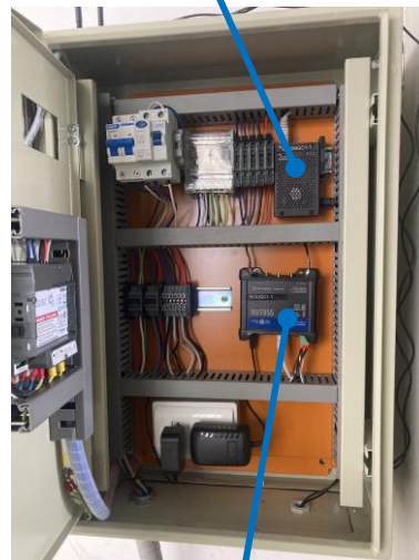
Router Teltonika/RUT955
